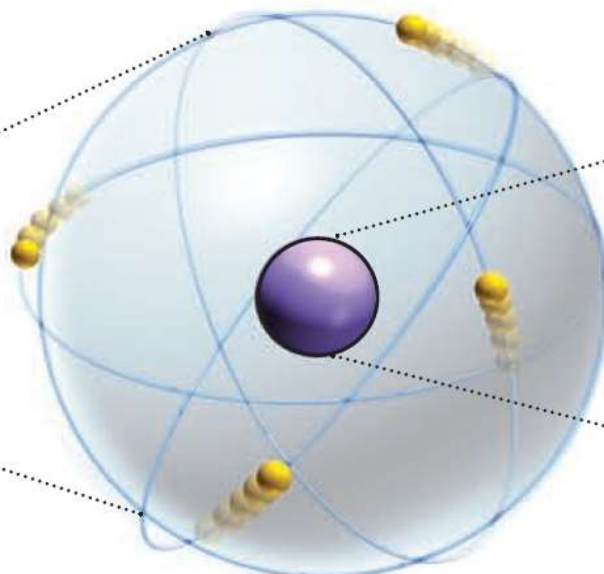
原子
