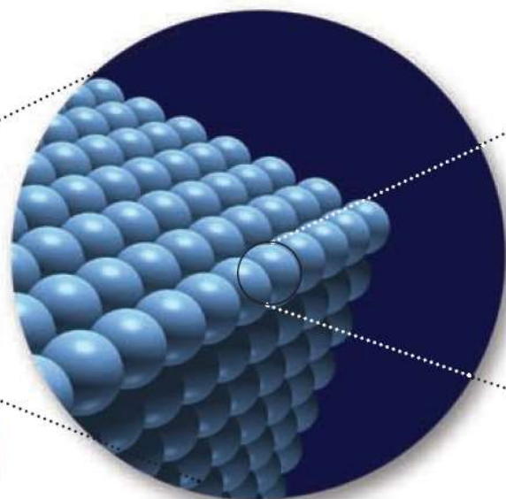
物質
