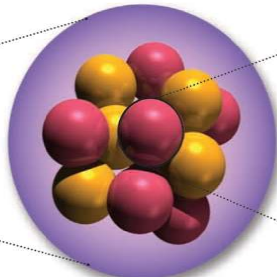
原子核
